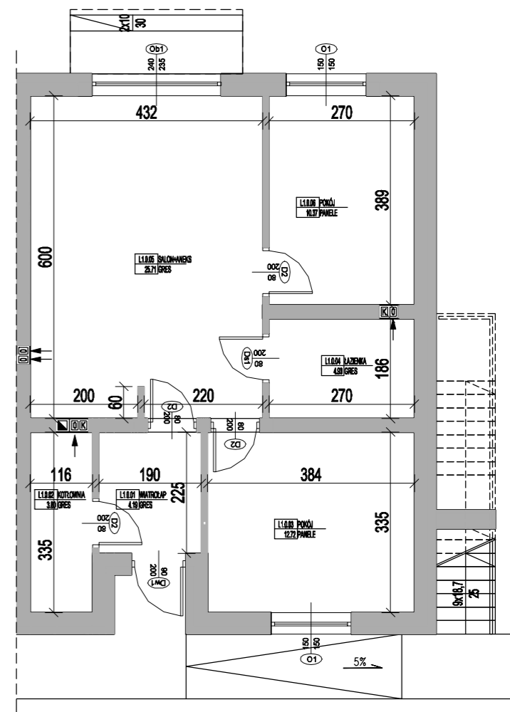
RZUT PARTERU
