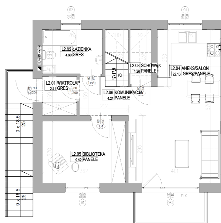
RZUT PARTERU
