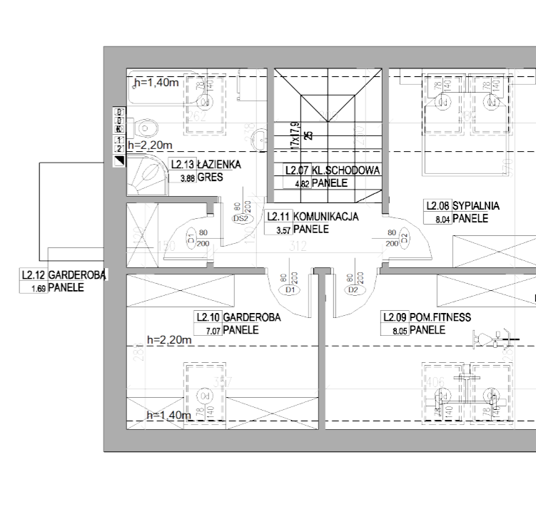
RZUT PODDASZA
