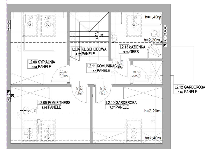
RZUT PODDASZA
