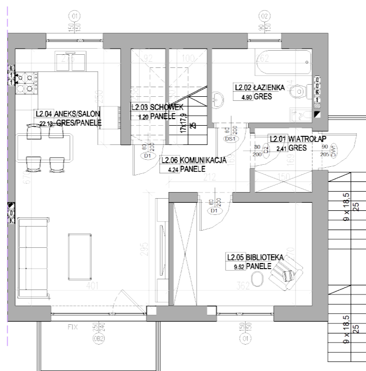
RZUT PARTERU
