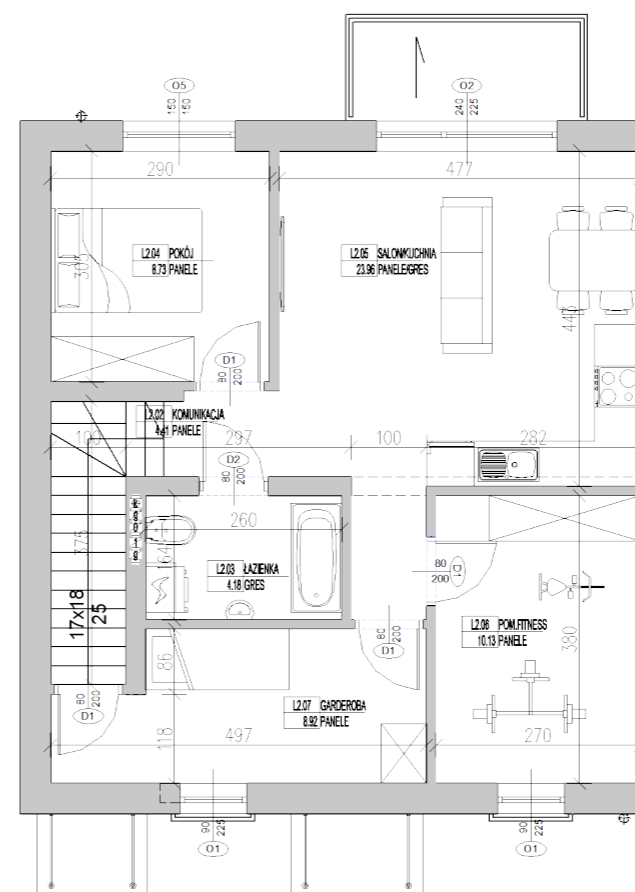
RZUT PIĘTRA
