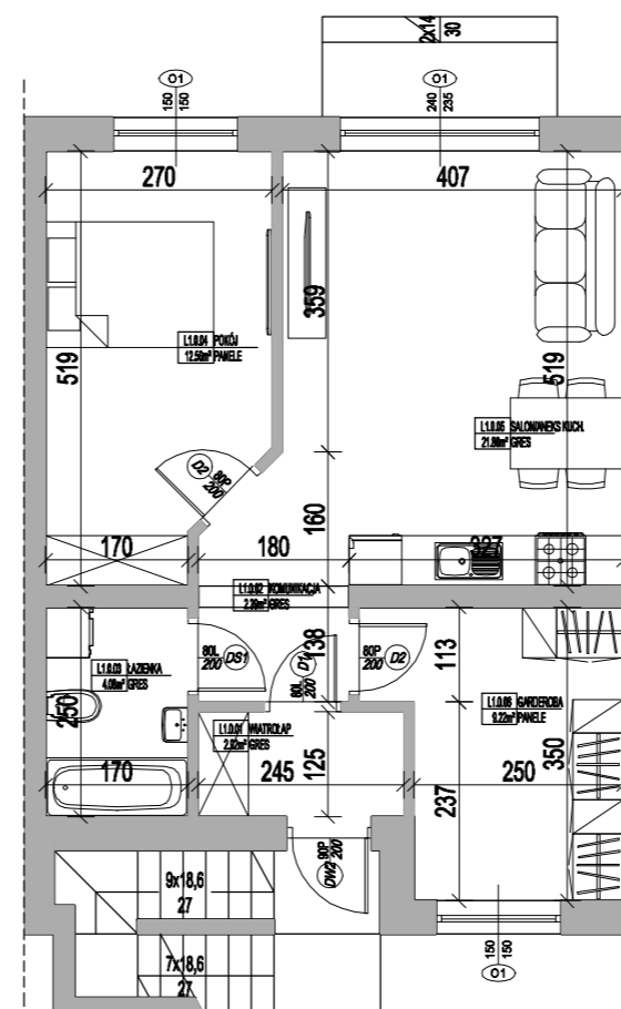
RZUT PARTERU
