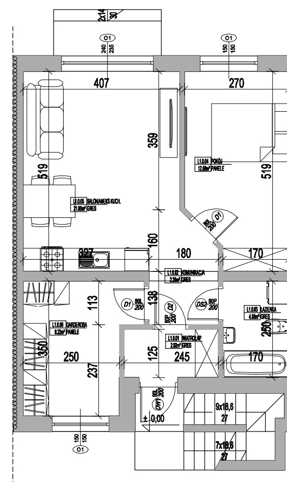
RZUT PARTERU
