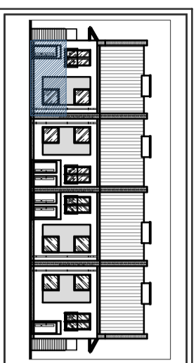
ELEWACJA FRONTOWA
