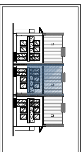
ELEWACJA OGRODOWA
