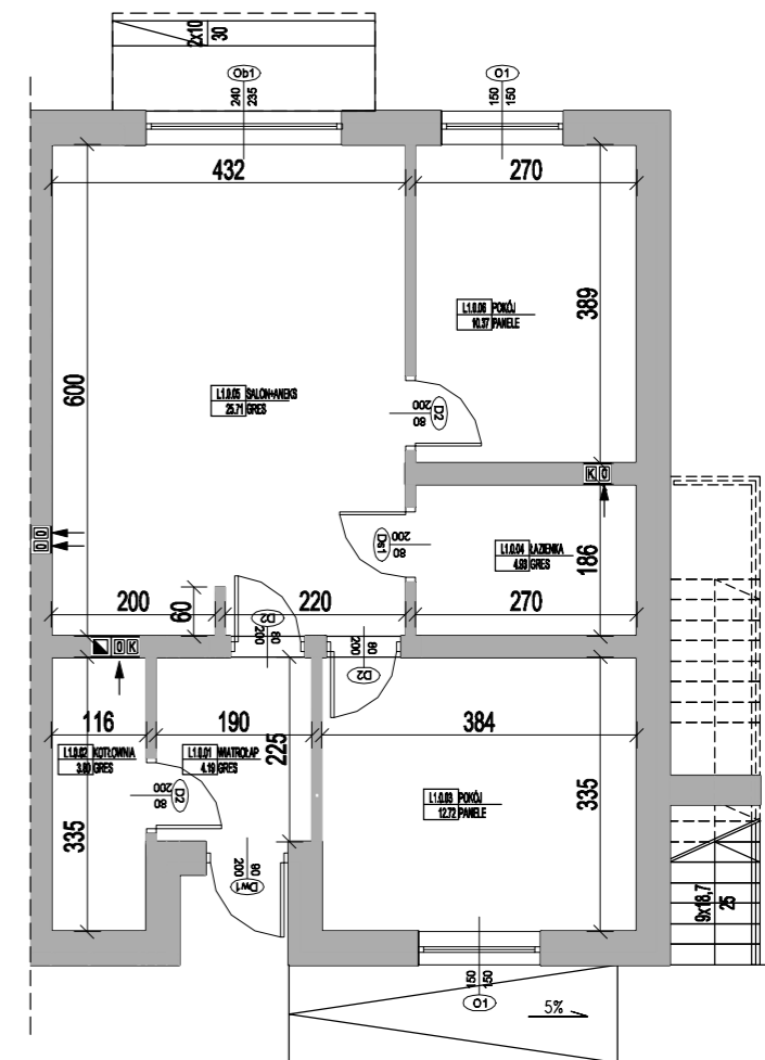
RZUT PARTERU
