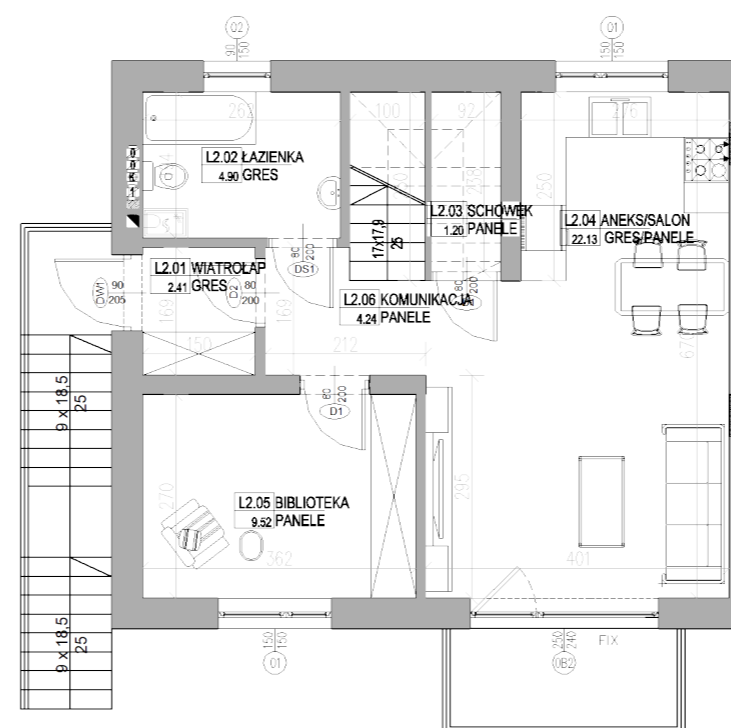
RZUT PARTERU
