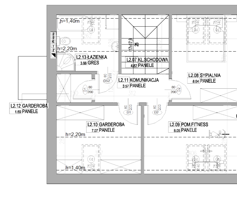
RZUT PODDASZA
