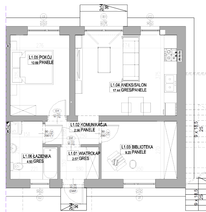
RZUT PARTERU
