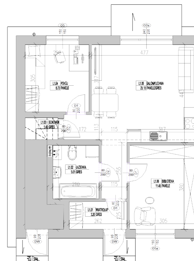
RZUT PARTERU
